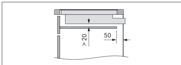
Afb. 5.2 Zijaanzicht inlegbodem voor kabelbescherming en verluchting
