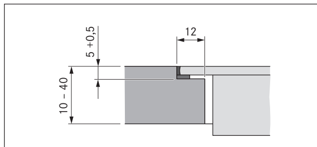
Afb. 5.4 Snede voegmaat
