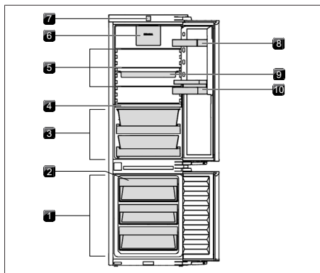
Fig. 5.4 Struttura C178KGW
