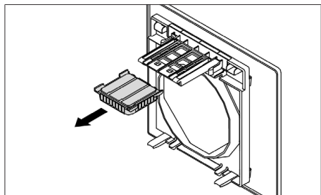
Fig. 10.2 Rimuovere il filtro antiodori
