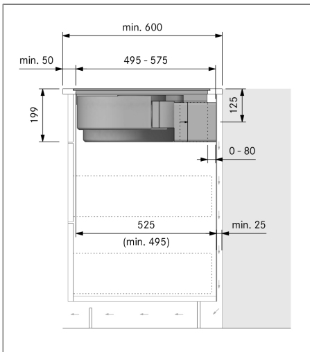
Fig. 9.21 Dimensioni di montaggio con sistema filtrante, variante di montaggio A
