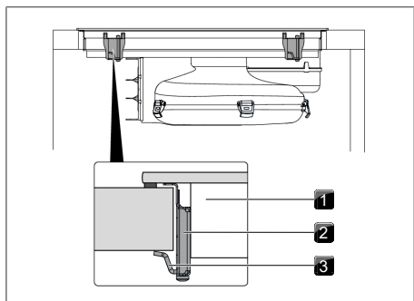
Fig. 9.31 Fissare il piano cottura nel centro
