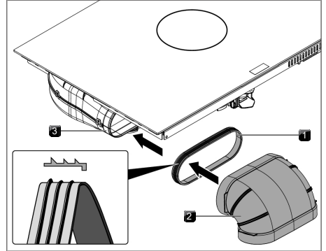
Fig. 9.17 Connessione al sistema di canali
