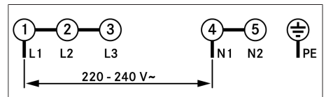
Fig. 9.35 Schema di collegamento collegamento monofase
