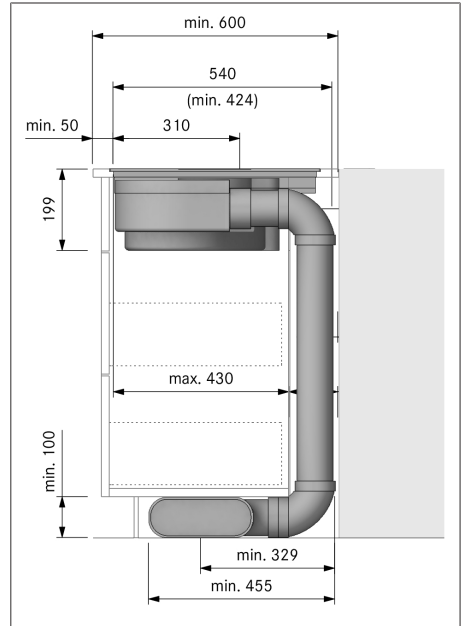
Fig. 9.9 Dimensioni di montaggio con sistema aspirante, profondità piano di lavoro 600 \text{ mm}
