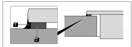
Fig. 9.10 Nastro a tenuta per montaggio in battuta
