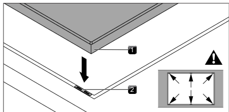
Fig. 9.29 Posizionamento dei pannelli di compensazione altezza
