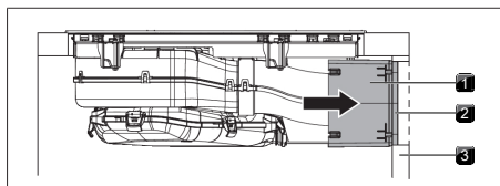
Fig. 9.32 Connessione parete posteriore
