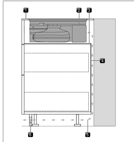
Fig. 9.19 Variante de montaje con base intermedia
