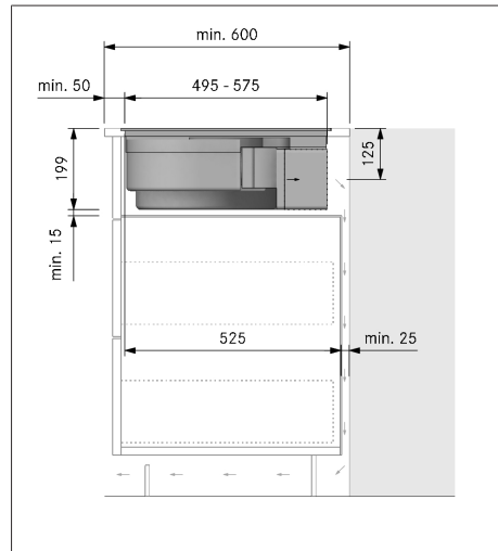
Fig. 9.23 Medidas de montaje para la variante de recirculación B, profundidad de la encimera 600 mm
