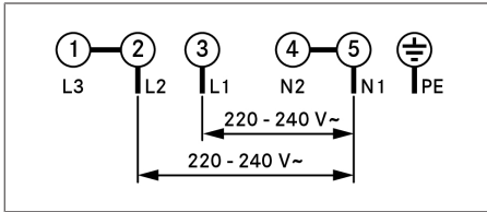
Fig. 9.39 Esquema de conexiones, conexión bifásica
