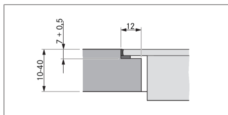
Fig. 9.8 Medida del rebaje para un montaje enrasado
