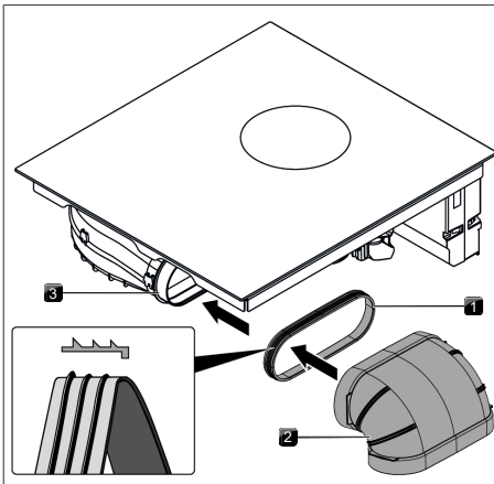
Fig. 9.16 Conexión al sistema de conductos
