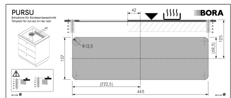
Fig. 9.22 Plantilla para el recorte del panel trasero
