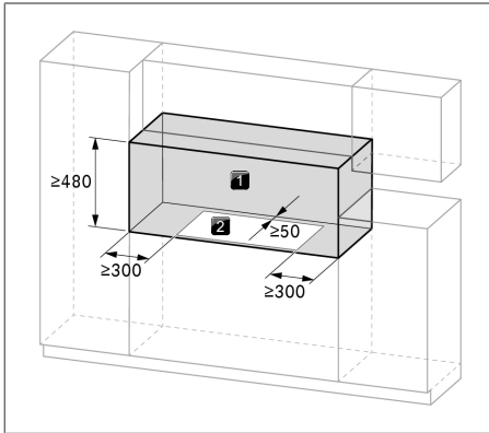
Fig. 9.3 Espacio libre requerido
