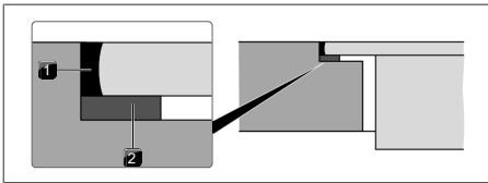
Fig. 9.25 Cinta selladora para montaje enrasado
