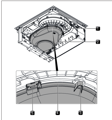
Fig. 7.3 Carcasa de conducción del aire
