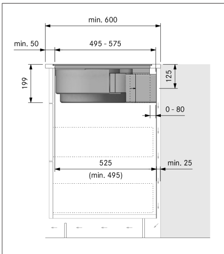
Fig. 9.20 Medidas de montaje con recirculación, variante de montaje A
