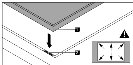
Fig. 9.28 Colocación de placas de compensación de altura
