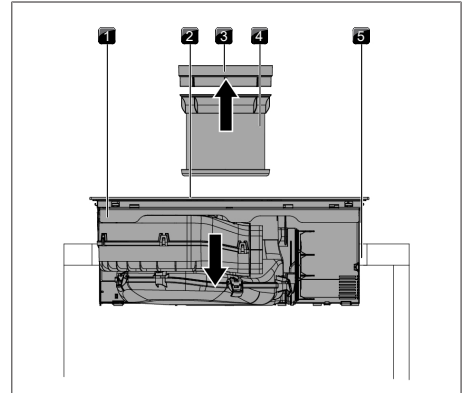
Fig. 9.26 Colocación de la placa de cocción
