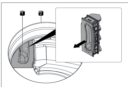
Fig. 9.31 Retirar la trampilla para el cambio del filtro
