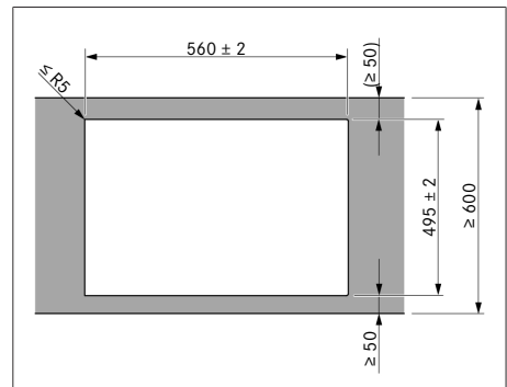
Fig. 9.5 Medidas del recorte para montaje superpuesto
