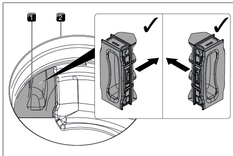
Fig. 7.10 Colocación de la trampa para el cambio del filtro
