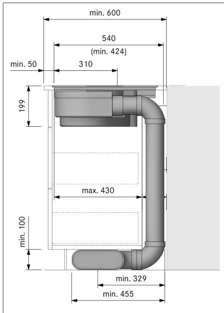
Fig. 9.9 Medidas de montaje para extracción al exterior, profundidad de la encimera 600 mm
