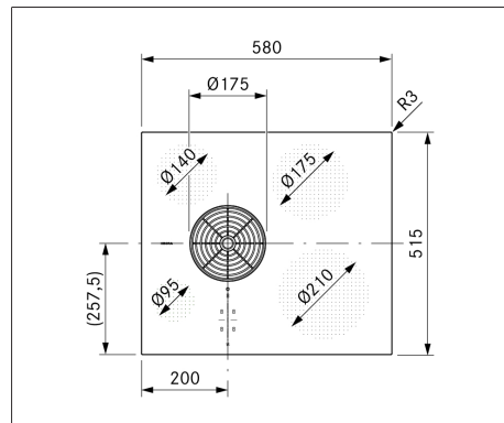
Fig. 3.1 Vista superior PURSA
