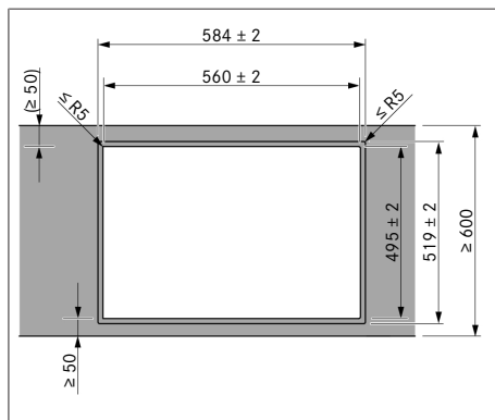
Fig. 9.7 Medidas del recorte para montaje enrasado
