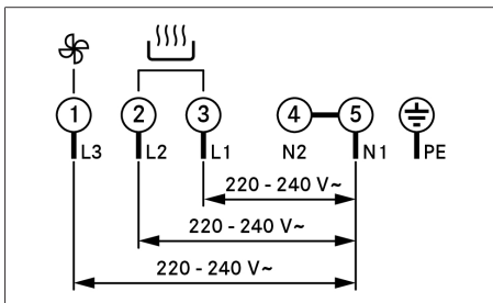
Fig. 9.38 Esquema de conexiones, conexión trifásica
