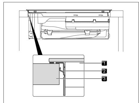
Fig. 9.27 Fijación de la placa de cocción
