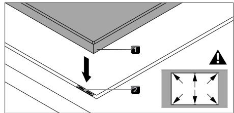
Fig. 9.14 Ubicación de placas de compensación de altura
