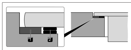
Fig. 9.29 Placas de compensación de altura
