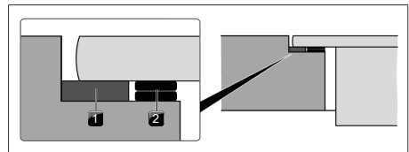
Fig. 9.15 Placas de compensación de altura
