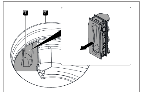
Fig. 9.35 Retirar la trampa para el cambio del filtro
