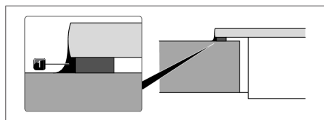
Fig. 9.47 Silicona de sellado para montaje superpuesto
