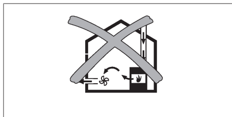
Fig. 9.1 Instalación de la extracción al exterior - no admisible
