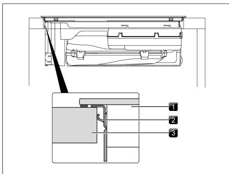
Fig. 9.13 Fijación de la placa de cocción en posición centrada
