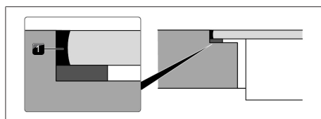
Fig. 9.48 Silicona de sellado para montaje enrasado
