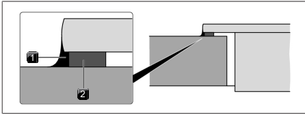
Fig. 9.24 Cinta selladora para montaje superpuesto
