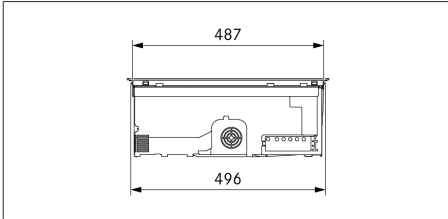
Fig. 3.3 Vista lateral PURSA
