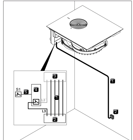
Fig. 9.42 Esquema de conexiones con contactos de conmutación externos
