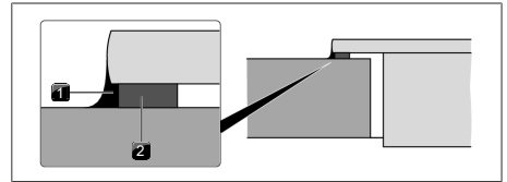
Fig. 9.10 Cinta selladora para montaje superpuesto
