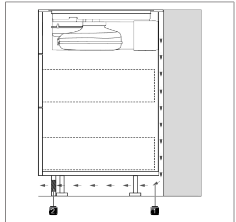
Fig. 9.17 Abertura de flujo de retorno en la zona del zócalo
