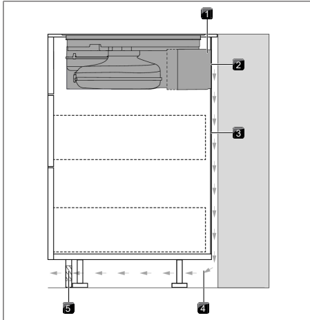
Fig. 9.18 Variante de montaje con panel trasero continuo
