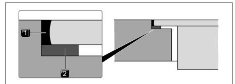
Fig. 9.11 Cinta selladora para montaje enrasado
