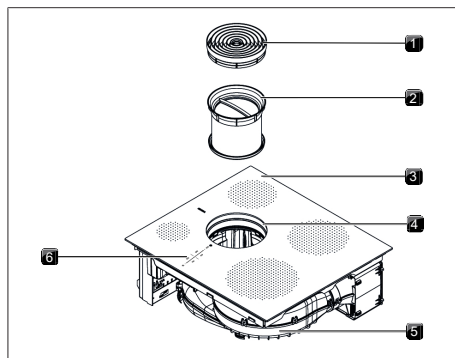
Fig. 4.1 Placa de cocción
