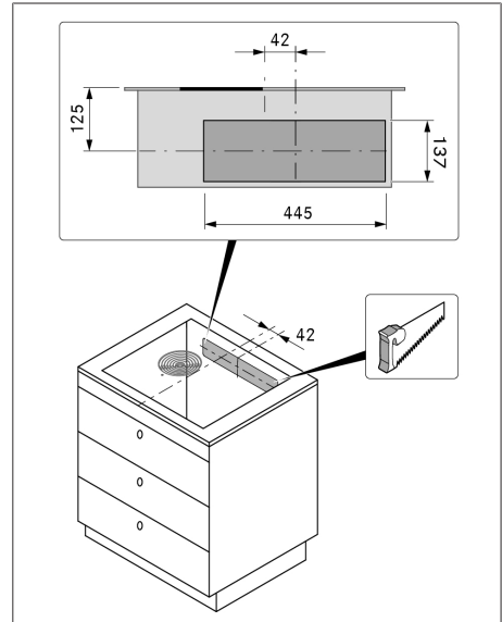
Fig. 9.21 Recorte del panel trasero
