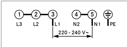
Fig. 9.40 Esquema de conexiones conexión monofásica
