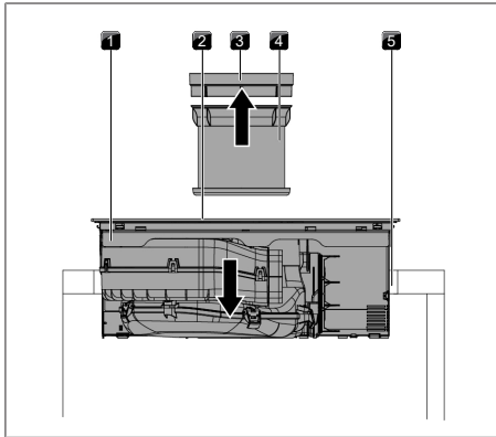
Fig. 9.12 Colocación de la placa de cocción
