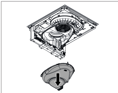
Fig. 9.37 Desmontaje de la parte inferior del espacio de aspiración
