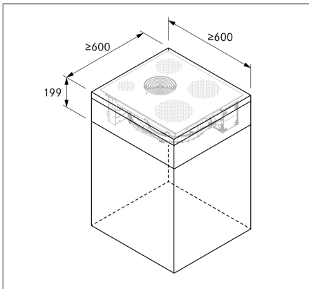
Fig. 9.4 Medidas mínimas de los muebles S Pure
