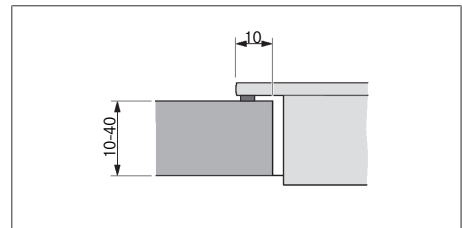
Fig. 9.6 Medida del apoyo para montaje superpuesto
