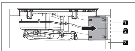
Fig. 9.30 Conexión del panel trasero
