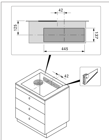
Fig. 9.21 Découpe dans la paroi arrière
