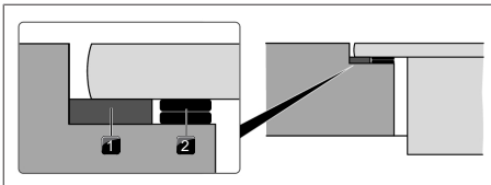
Fig. 9.29 Plaques de compensation des hauteurs
