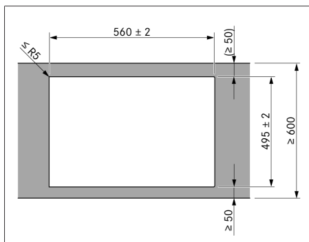
Fig. 9.5 Dimensions de découpe pour montage en saillie
