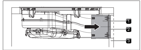
Fig. 9.30 Raccordement à la paroi arrière
