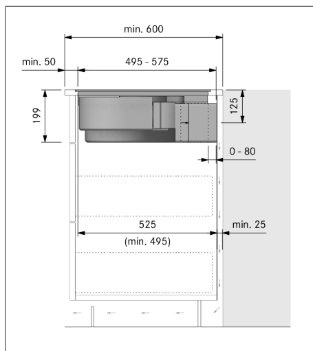
Fig. 9.20 Cotes de montage pour le recyclage d'air, variante A
