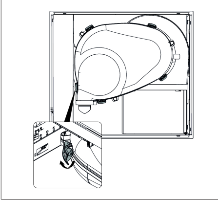
Fig. 9.36 Loquets du carter d'aspiration
