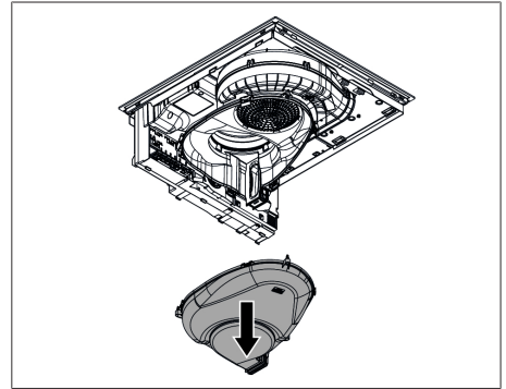
Fig. 9.37 Démontage du carter d'aspiration
