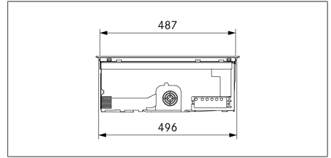
Fig. 3.6 Vue de côté PURSU
