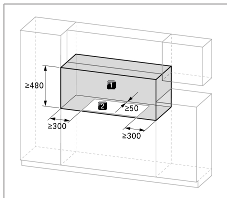
Fig. 9.3 Espace requis
