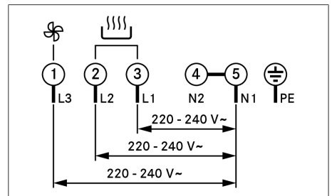
Fig. 9.38 Schéma de raccordement triphasé
