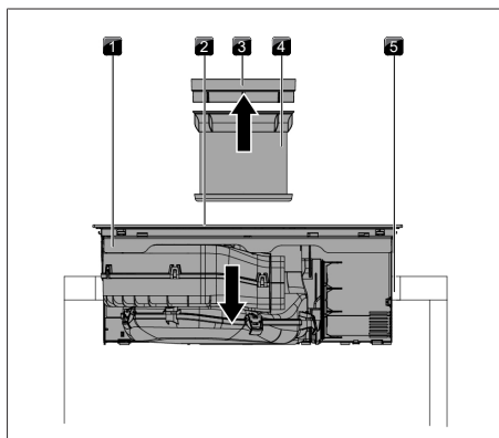
Fig. 9.26 Placer la table de cuisson
