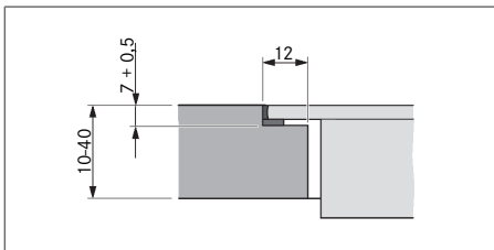
Fig. 9.8 Dimension de rainure pour montage affleurant
