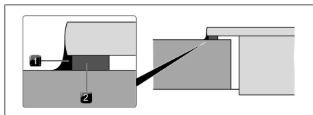
Fig. 9.24 Ruban d'étanchéité pour montage en saillie
