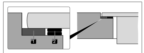
Fig. 9.15 Plaques de compensation des hauteurs
