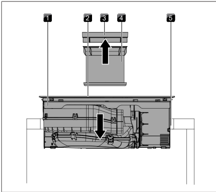
Fig. 9.12 Placer la table de cuisson
