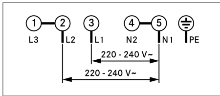
Fig. 9.39 Schéma de raccordement biphasé
