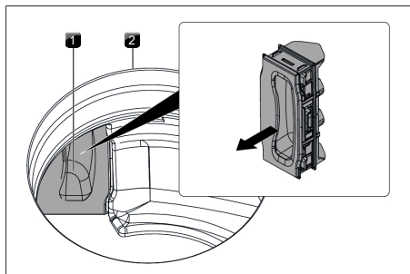
Fig. 9.35 Retrait du clapet de changement de filtre
