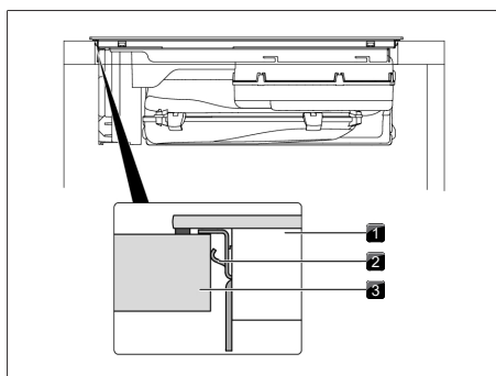
Fig. 9.27 Fixation de la table de cuisson
