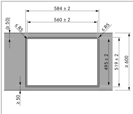
Fig. 9.7 Dimensions de découpe pour montage affleurant
