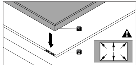
Fig. 9.14 Positionnement des plaques de compensation des hauteurs
