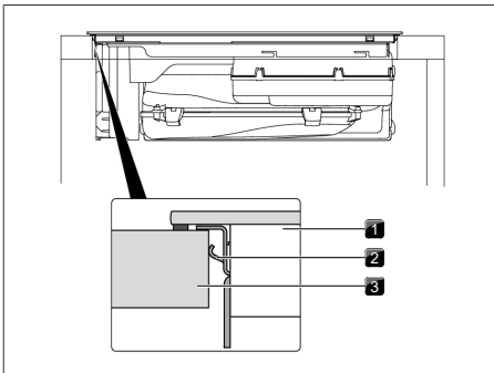
Fig. 9.13 Centrage et fixation de la table de cuisson
