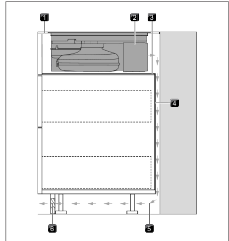
Fig. 9.19 Variante de montage avec fond intermédiaire
