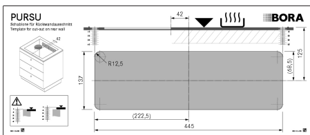
Fig. 9.22 Gabarit de découpe dans la paroi arrière
