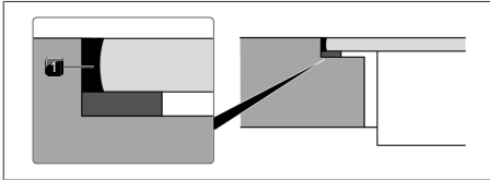
Fig. 9.48 Joint en silicone en montage affleurant
