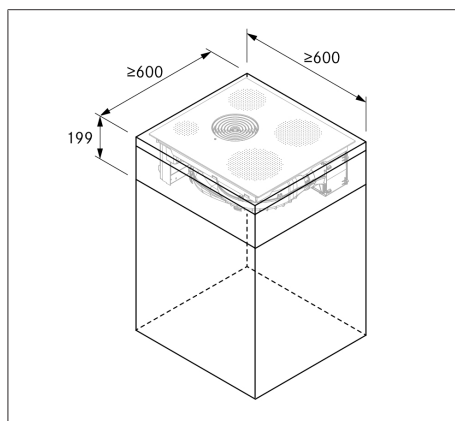
Fig. 9.4 Dimensions minimales du meuble pour S Pure
