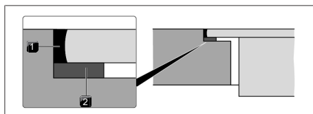
Fig. 9.25 Ruban d'étanchéité pour montage affleurant
