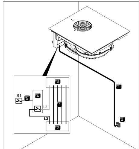
Fig. 9.42 Schéma de raccordement avec contacts externes
