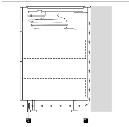
Fig. 9.17 Ouverture de retour de flux dans le socle
