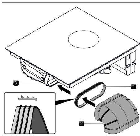
Fig. 9.16 Raccordement au système de canaux
