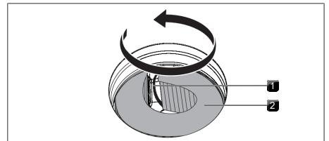
Fig. 7.5 Retrait du filtre à charbon actif de son boîtier
