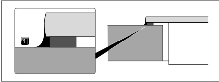
Fig. 9.47 Joint en silicone en montage en saillie
