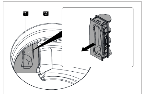
Fig. 9.31 Retrait du clapet de changement de filtre
