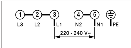
Fig. 9.40 Schéma de raccordement monophasé
