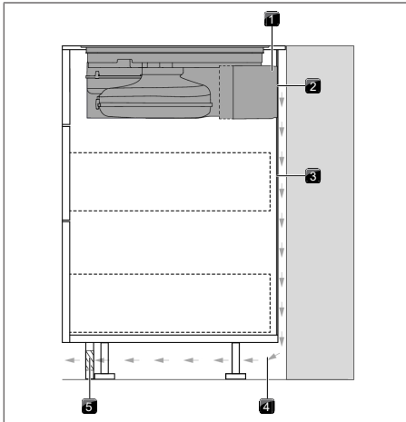
Fig. 9.18 Variante de montage avec paroi arrière intégrale
