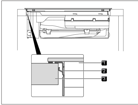
Kuva 9.13 Keittotason kiinnittäminen keskelle
