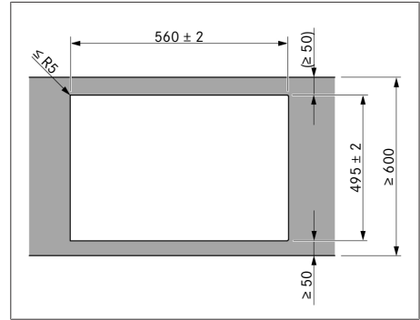
Kuva 9.5 Asennusaukkojen mitat pinta-asennusta varten
