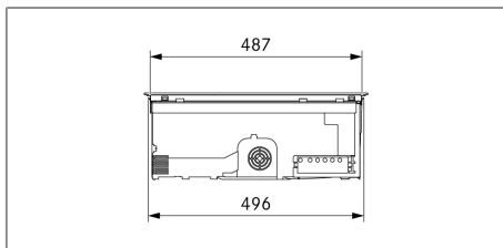
Kuva 3.3 PURSA, sivukuva
