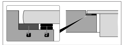
Kuva 9.29 Korkeussäätölevyt
