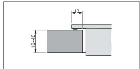
Kuva 9.6 Alustan mitat pinta-asennusta varten
