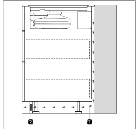
Kuva 9.17 Paluuilman aukko sokkelialueella
