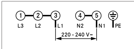
Kuva 9.40 Liitäntäkaavio - 1-vaiheiliitäntä
