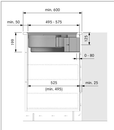
Kuva 9.20 Asennusmitat kiertoilmakäytössä, asennusvaihtoehto A
