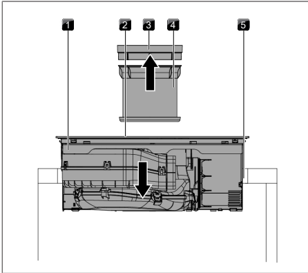
Kuva 9.26 Keittotason asettaminen paikalleen
