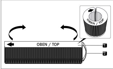
Kuva 7.7 Aktiivihiihisuodatin
