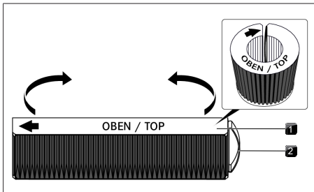
Kuva 9.32 Aktiivihiihisuodatin
