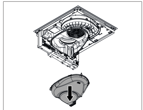
Kuva 9.37 Imutilan alaosan irrottaminen
