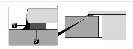
Kuva 9.10 Tiivistenauha pinta-asennuksessa
