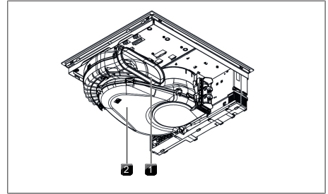
Kuva 4.2 Näkymä takaa PURSA
