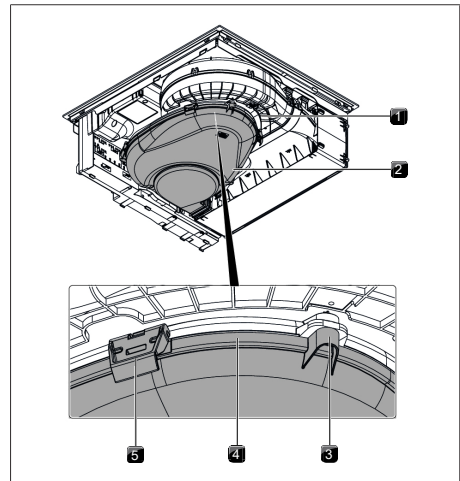
Kuva 7.3 Ilmanohjaukotelon
