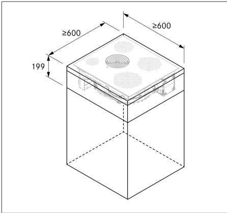
Kuva 9.4 Kalusteen vähimmäismitat S Pure
