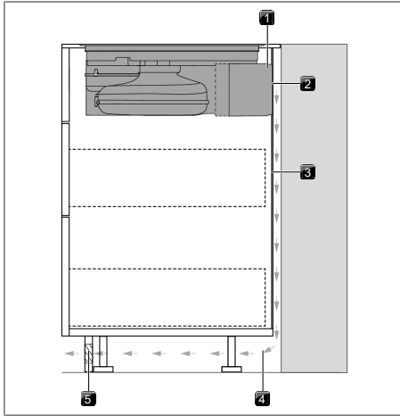
Kuva 9.18 Asennusvaihtoehto, jossa yhtenäinen takaseinä
