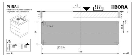
Kuva 9.22 Sapluuna takaseinän aukkoa varten
