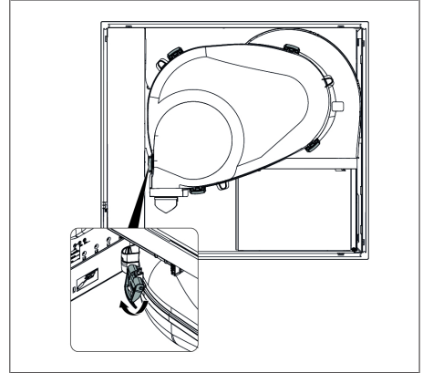
Kuva 9.36 Imutilan kiinnikkeet
