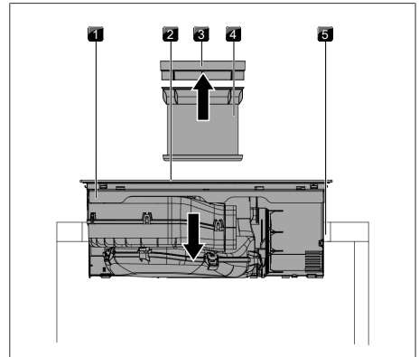
Kuva 9.12 Keittotason asettaminen paikalleen
