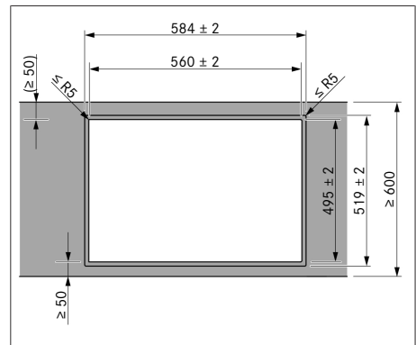
Kuva 9.7 Asennusaukkojen mitat uppoasennusta varten
