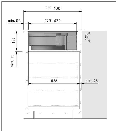
Kuva 9.23 Asennusmitat kiertoilma-asennuksessa B, työtason syvyys 600 mm
