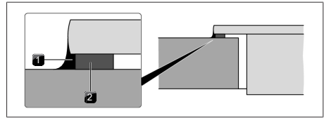
Kuva 9.24 Tiivistenuaha pinta-asennuksessa
