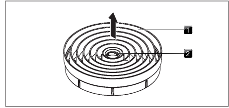
Kuva 7.1 Höyrypoistoritilän irrottaminen
