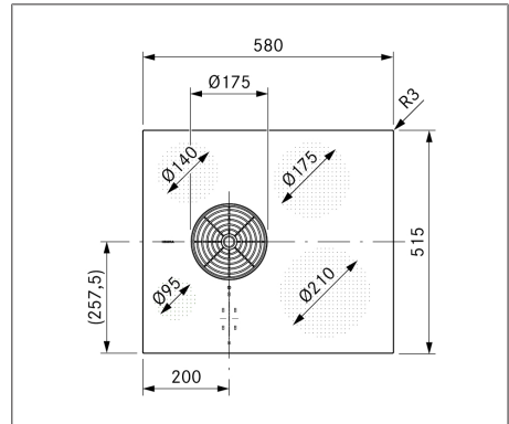
Kuva 3.1 PURSA, kuva ylhäältä
