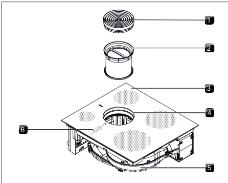
Kuva 4.1 Keittotasoa
