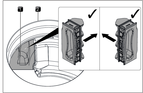
Kuva 7.10 Suodattimen vaihtoläpän asettaminen
