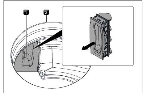
Kuva 7.4 Suodattimen vaihtoläppän irrottaminen
