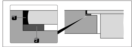
Kuva 9.25 Tiivistenuaha uppoasennuksessa
