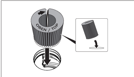
Kuva 7.8 Aktiivihiihisuodattimen asettaminen tuloaukkoon
