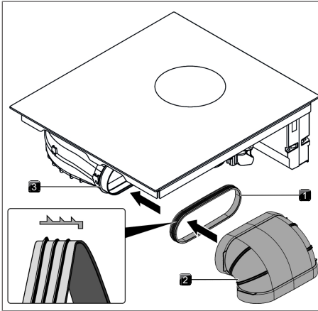
Kuva 9.16 Liittäminen kanavajärjestelmään
