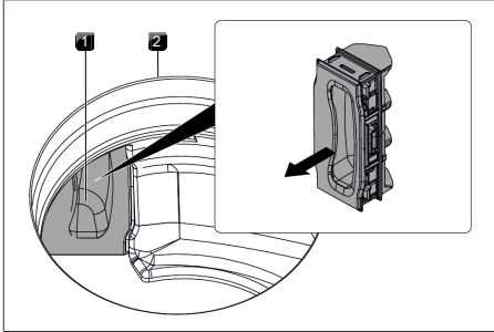
Kuva 9.35 Suodattimen vaihtoläpän irrottaminen
