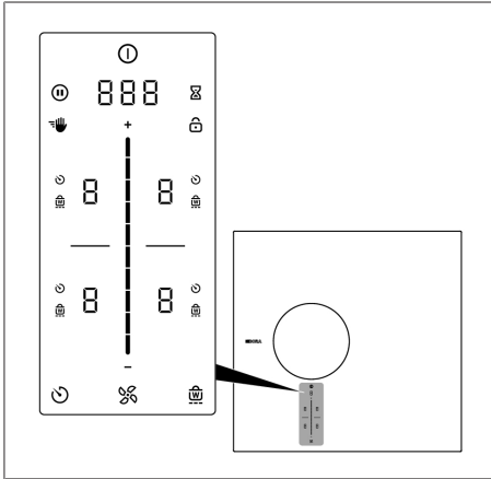
Kuva 4.4 Keskeillä oleva hipaisu-/liikusäädinpaneeli
