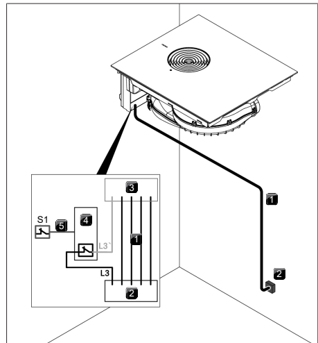
Kuva 9.42 Liitäntäkaavio, ulkoiset kytkimet
