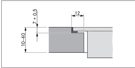
Kuva 9.8 Saumamitta uppoasennusta varten
