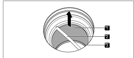
Kuva 7.2 Ruostumattomasta teräksestä valmistetun rasvasuodattimen irrottaminen
