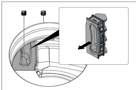
Kuva 9.31 Suodattimen vaihtoläpän irrottaminen
