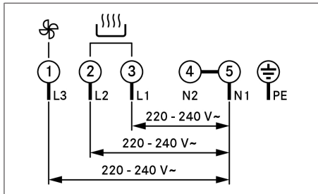
Kuva 9.38 Liitäntäkaavio - 3-vaiheiliitäntä
