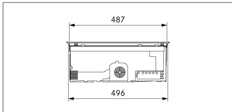
Kuva 3.6 PURSU, sivukuva
