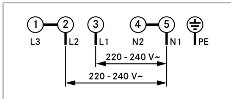
Kuva 9.39 Liitäntäkaavio - 2-vaiheiliitäntä
