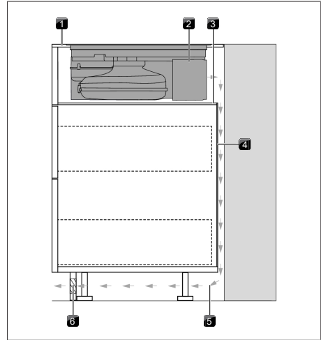
Kuva 9.19 Asennusvaihtoehto, jossa välipohja
