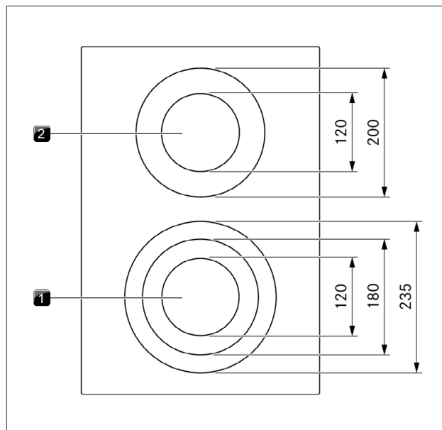
Fig. 3.11 Opbygning af kogeplade PKC3 og størrelse af kogezone
