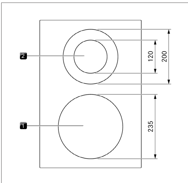
Fig. 3.13 Opbygning af kogeplade PKCH3 og størrelse af kogezone
