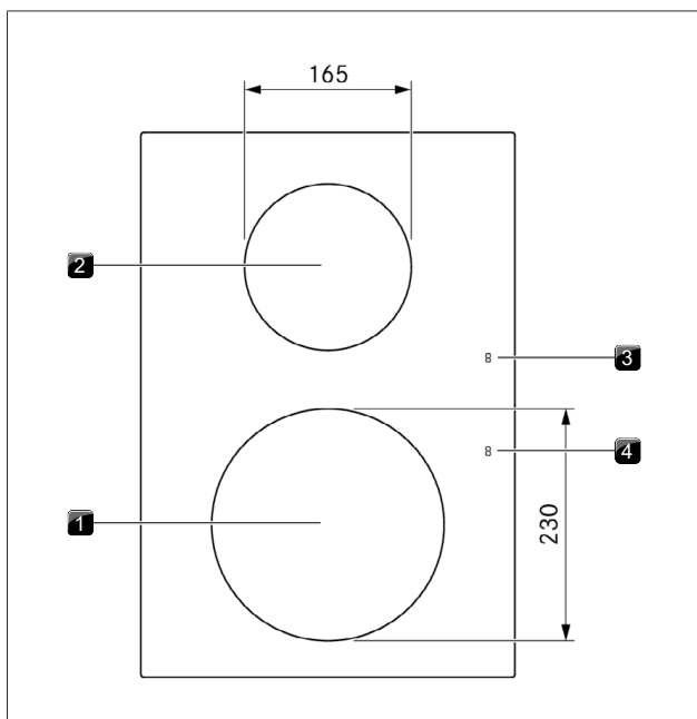
Fig. 3.9 Opbygning af kogeplade PKI3 og størrelse af kogezone
