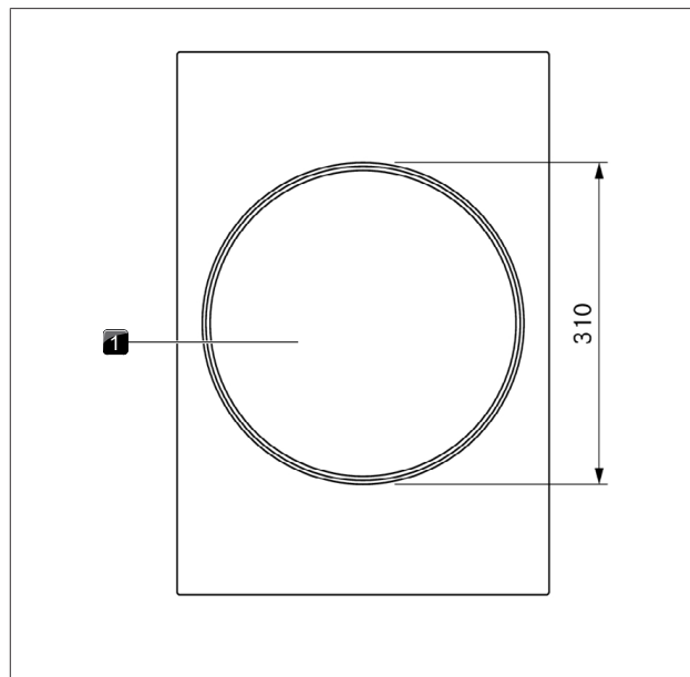
Fig. 3.10 Opbygning af kogeplade PKIW3 og størrelse af kogezone
