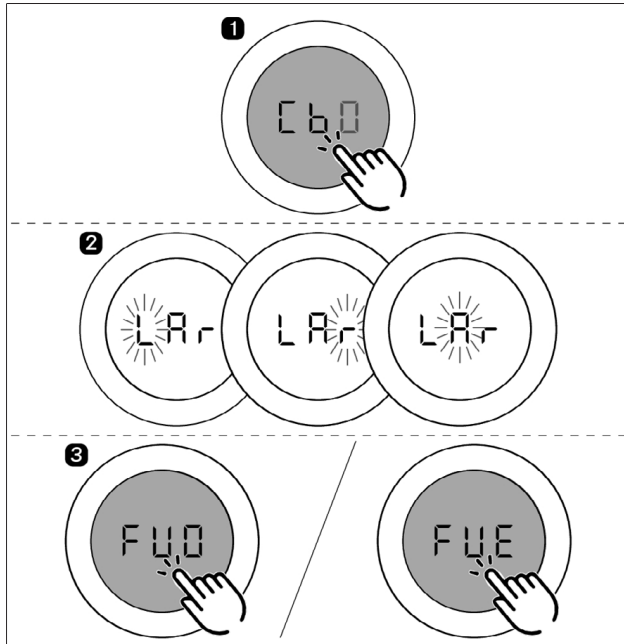
Fig. 6.6 Begynd softwareopdatering
