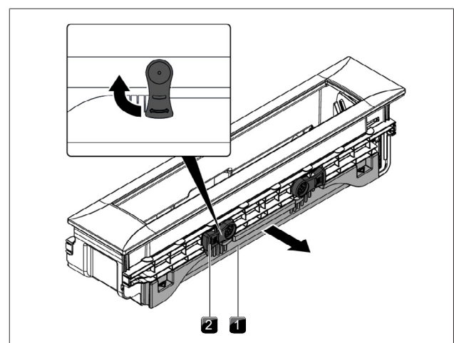
Fig. 7.4 Afmontering af vedligeholdelsesbakke
