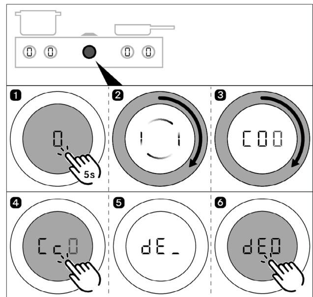
Fig. 6.7 Foretag dataeksport
