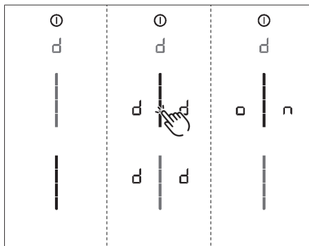
Fig. 9.50 Display Menu item D: Demo mode
